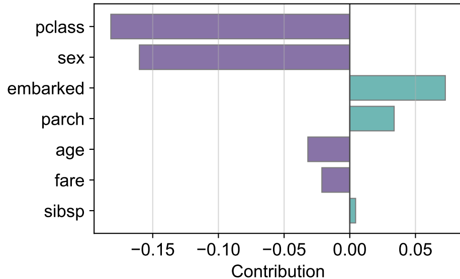
LIME
