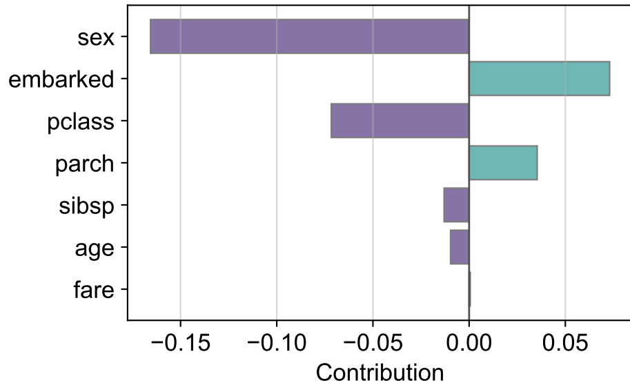
SHAP
